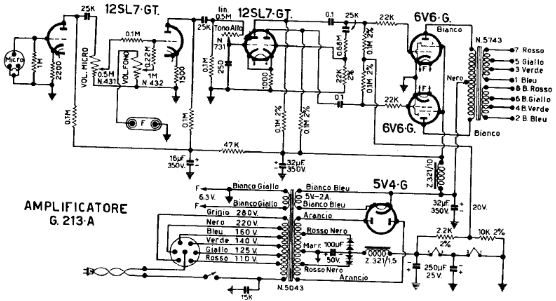
AMPLIFICATORE 12 ÷ 15 WATT B.F. - TIPO G 213 A
